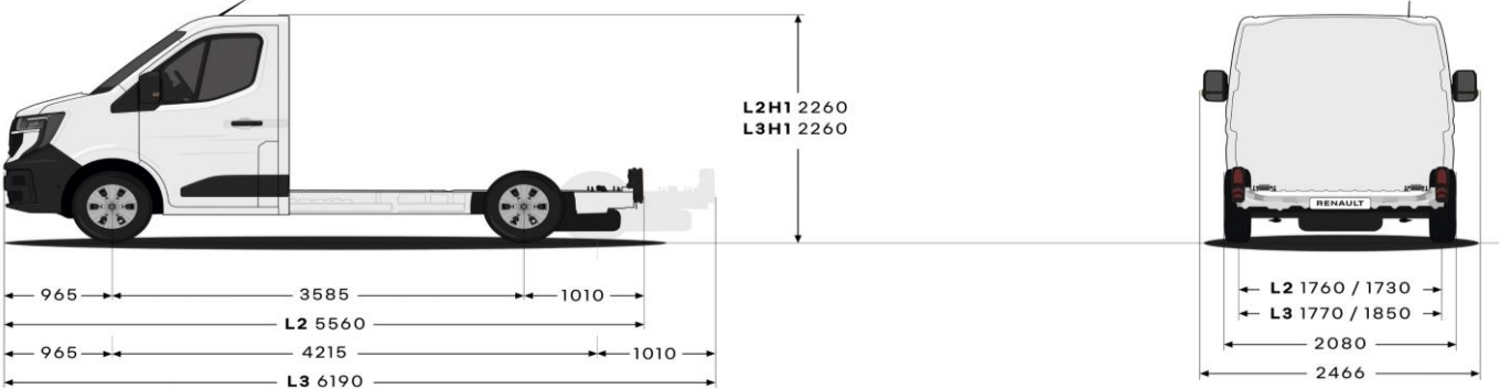
Chassi-platta enkelhytt (mått i mm)
