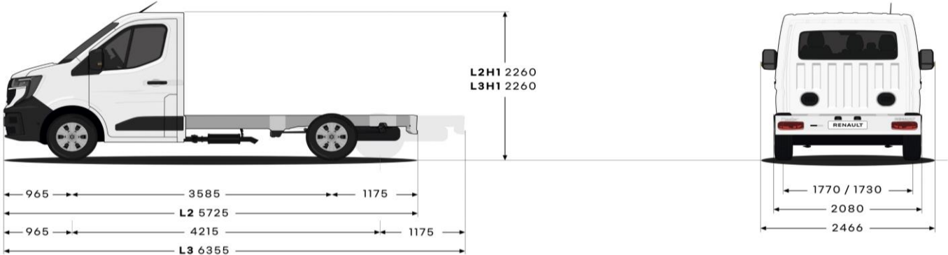
Chassi enkelhytt (mått i mm)
