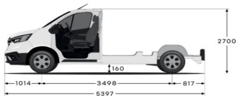
Chassi-platta
